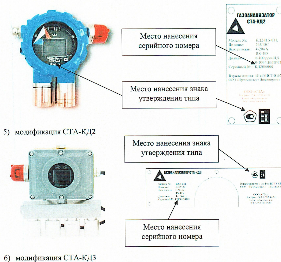
Рисунок 1 – Общий вид газоанализаторов
